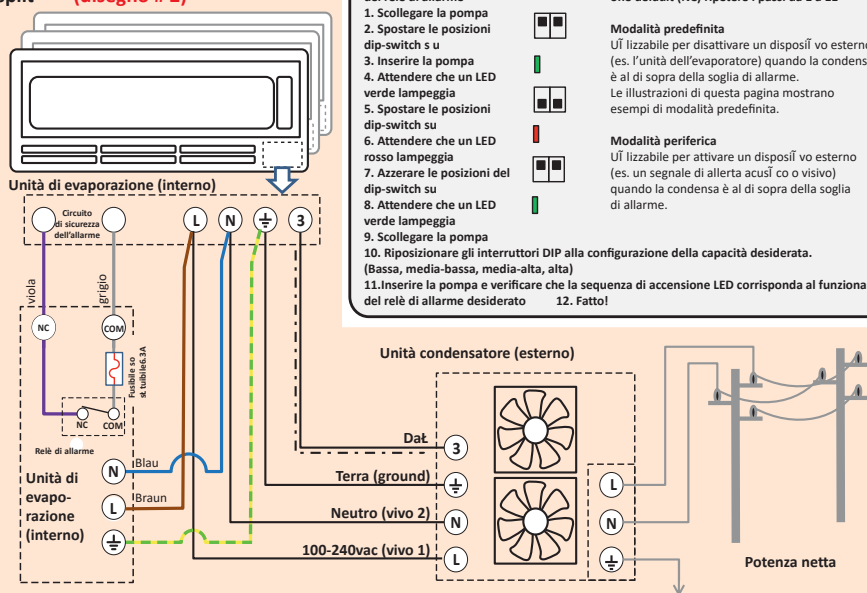
Quando è installato un sistema mult-split (disegno # 2)
